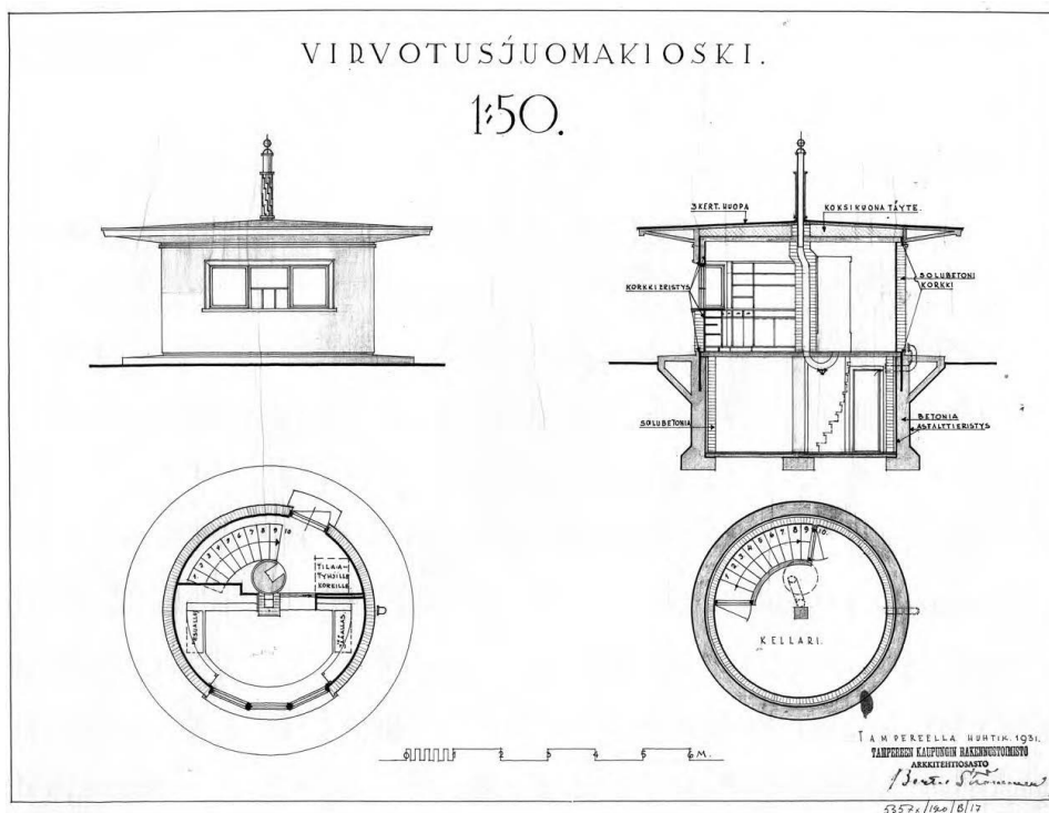
Bertel Strömmerin tyyppipiirustukset v. 1931; julkisivu, leikkaus ja pohjapiirrokset
