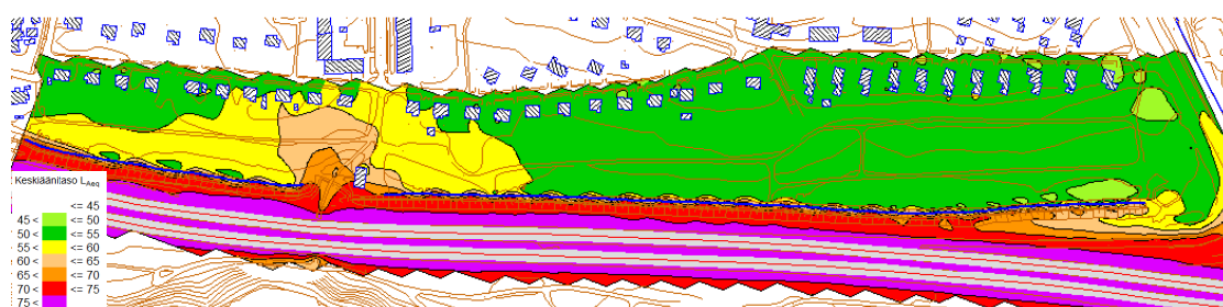
Kuva 12. Vuoden 2040 ennustetut päivämelualueet parannetulla meluntorjunnalla, kohde 72
