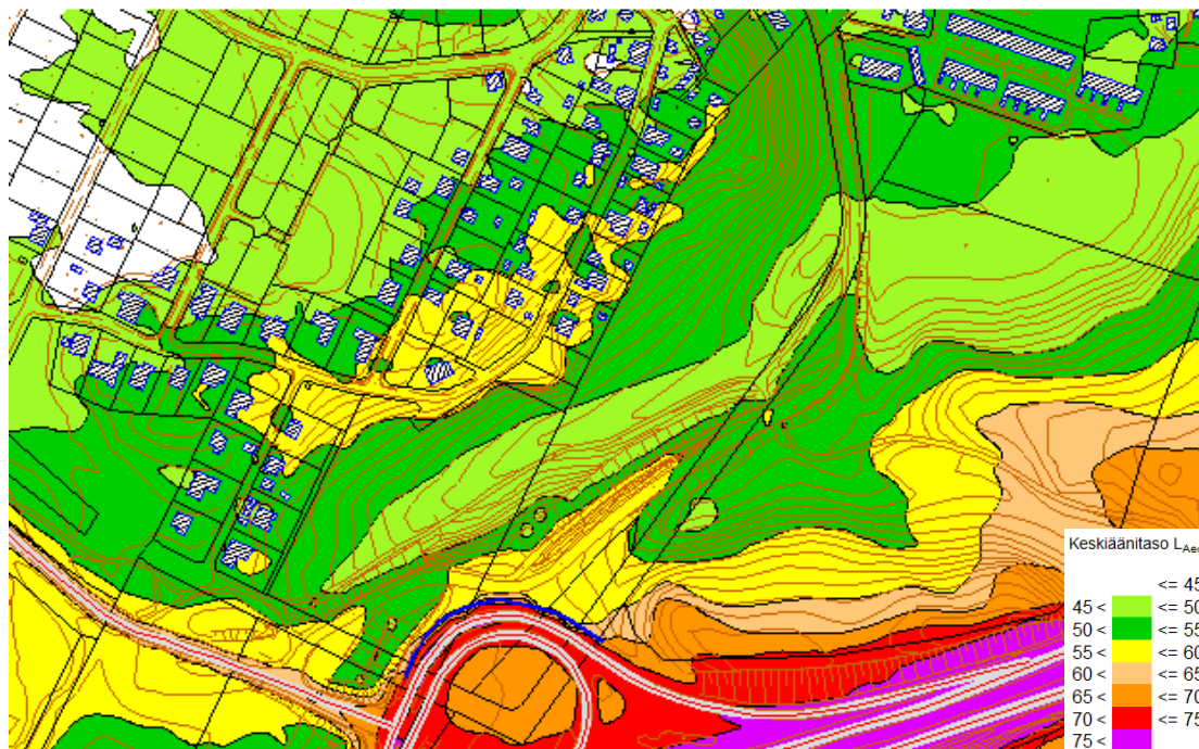
Kuva 3. Vuoden 2040 ennustetut päivämelualueet nykyisellä maankäytöllä, kohde 69
