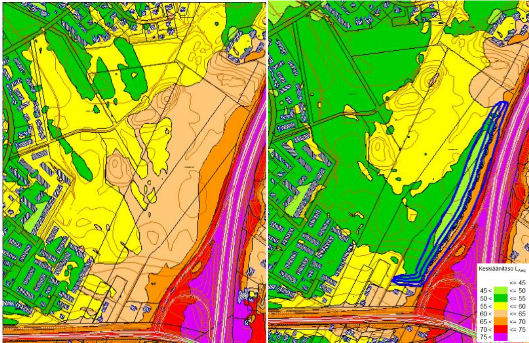
Kuva 8. Vuoden 2040 ennustetut päivämelualueet nykyisellä (kuvassa vasemmalla) ja parannetulla (kuvassa oikealla) meluntorjunnalla, kohde 45
