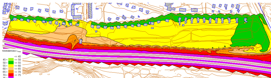
Kuva 11. Vuoden 2040 ennustetut päivämelualueet nykyisellä maankäytöllä, kohde 72
