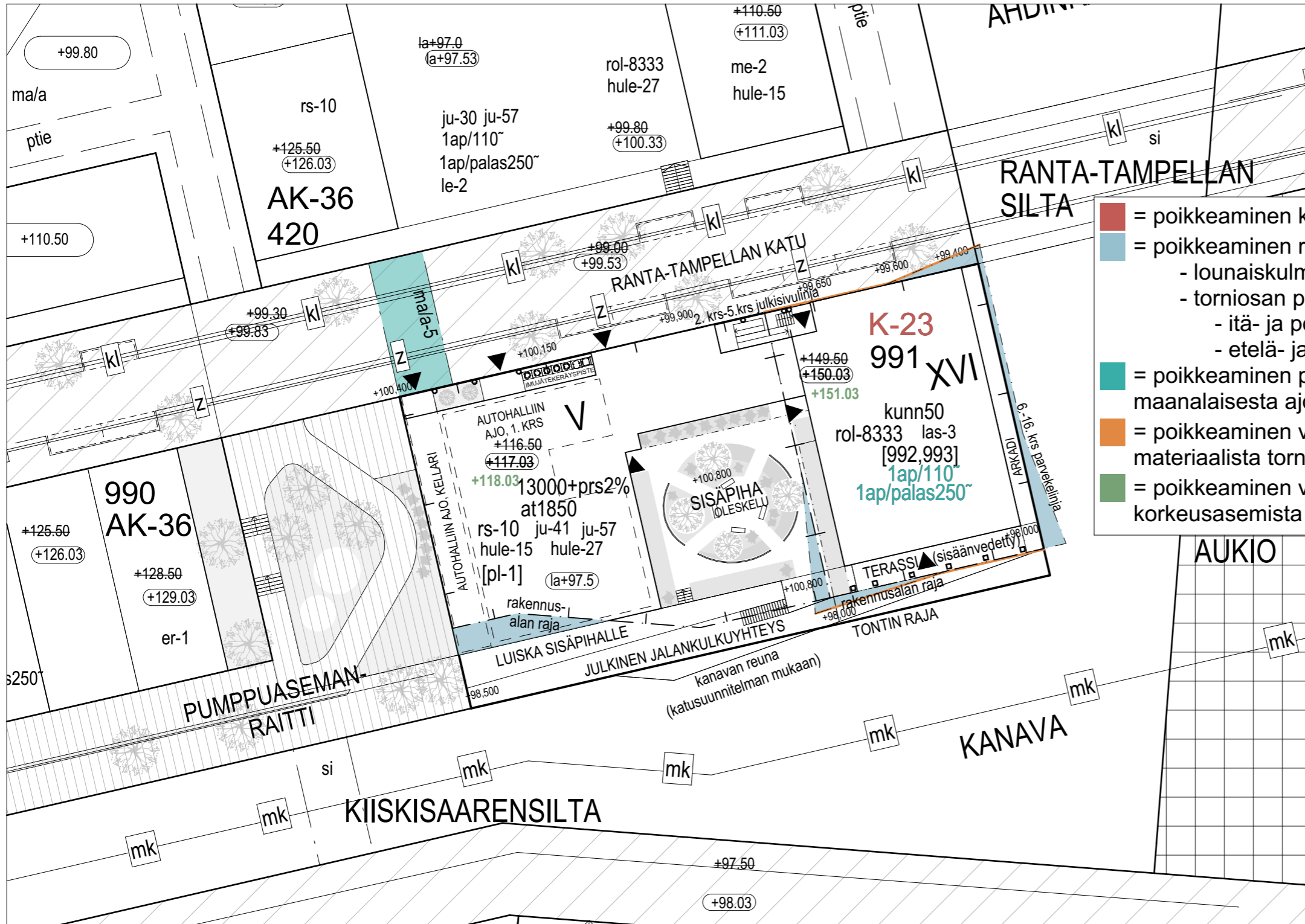
ASEMAPIIRROS 1:500 (POIKKEUKSILLA)
